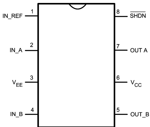
SOIC-8
